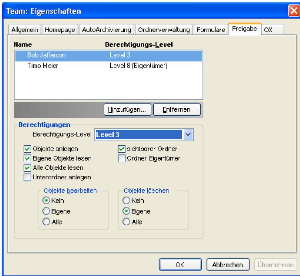
Abbildung 7.11. Berechtigungs-Level 3
